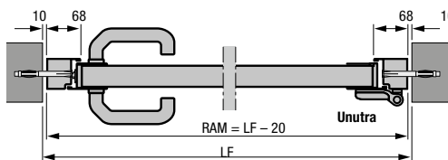
Bočna vrata sa aluminijumskim obuhvatnim štokom, tip profila 2 Ugradnja u otvor
