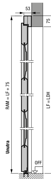
Bočna vrata od punog drveta Ugradnja iza otvora
