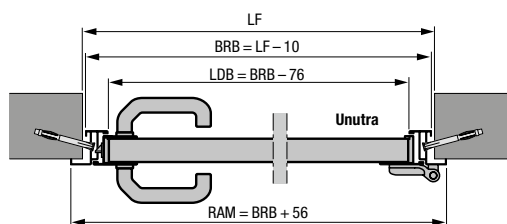
Bočna vrata sa aluminijumskim ugaonim štokom, tip profila 1 ili 2 Montaža sa unutrašnje strane
