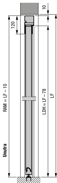
Bočna vrata sa aluminijumskim obuhvatnim štokom, tip profila 2 Ugradnja u otvor
