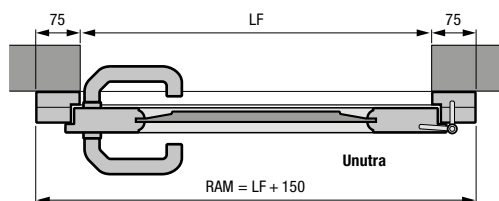
Bočna vrata od punog drveta Ugradnja iza otvora
