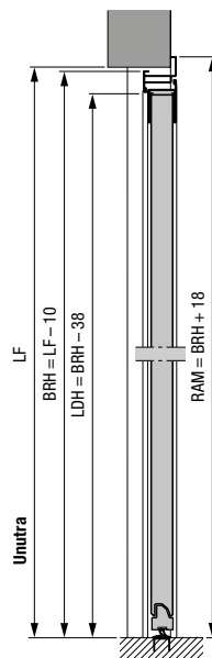
Bočna vrata sa aluminijumskim obuhvatnim štokom, tip profila 2 Sa spoljne strane
