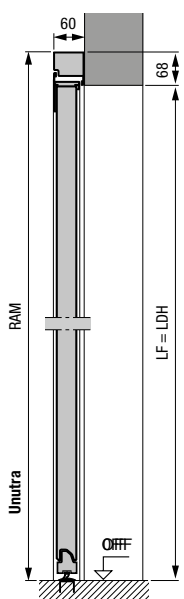
Bočna vrata sa aluminijumskim obuhvatnim štokom, tip profila 2 Ugradnja iza otvora
